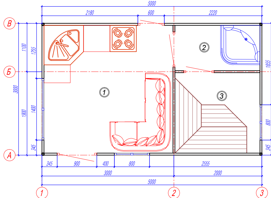
План
